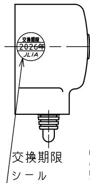
A矢視図
